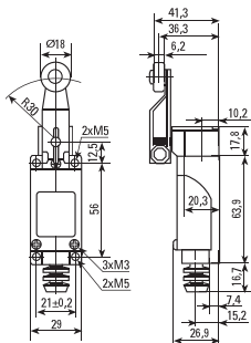
Рис. 1 - Габаритные размеры концевого выключателя TZ-8104
