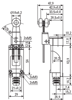
Рис. 2 - Габаритные размеры концевого выключателя TZ-8108
