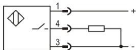
PNP NO
